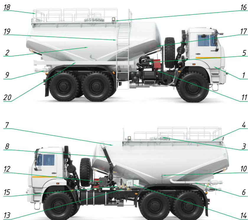
Рисунок 3 - Автоцементовоз АЦВ-17Р1-01.
